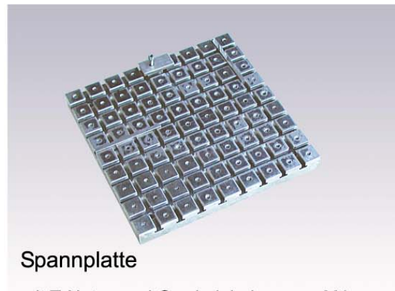
Aufnahme für 3 Fräsmotoren
